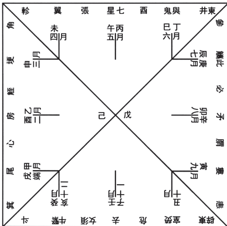
【図五】馬王堆帛書「陰陽五行甲篇」堪輿占図
