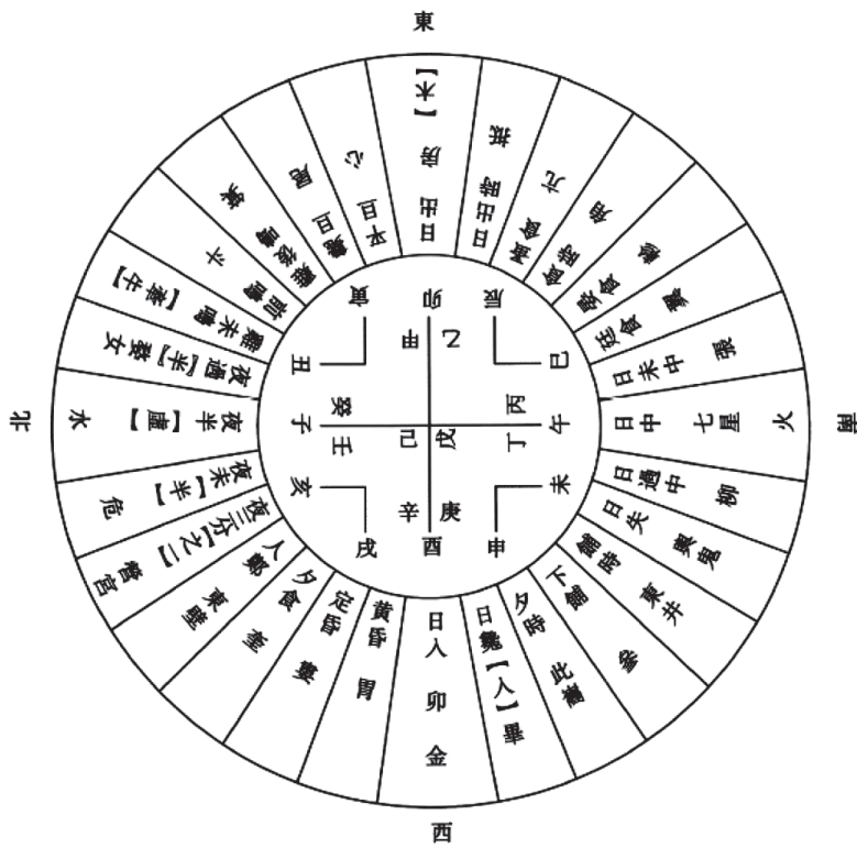
【図八】周家台秦簡「二十八宿占」式図
