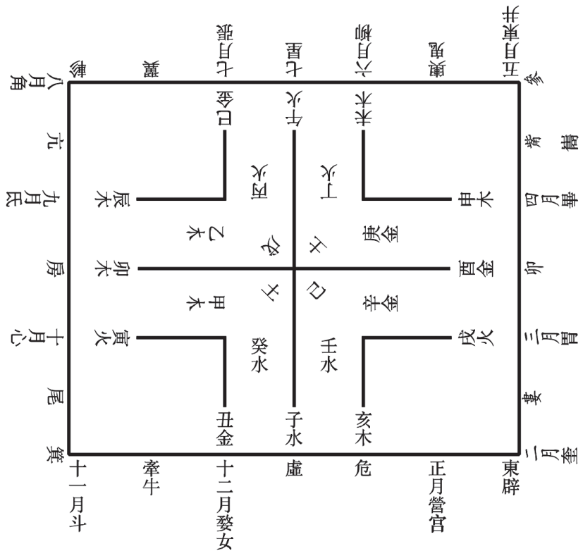
【図七】北大漢簡「日書・式図（乙）」
