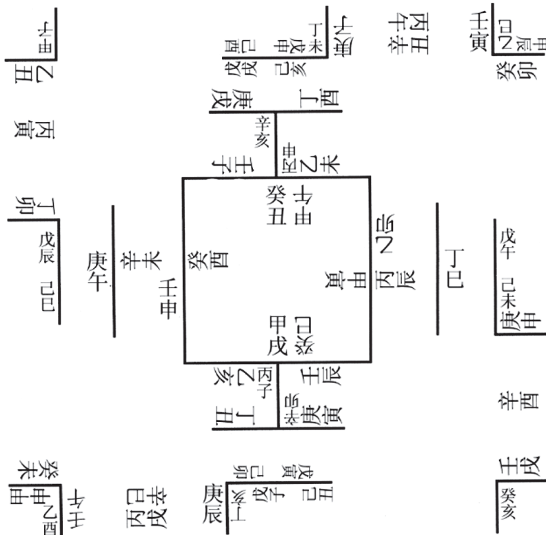
【図九】北大漢簡「六博」六博図
