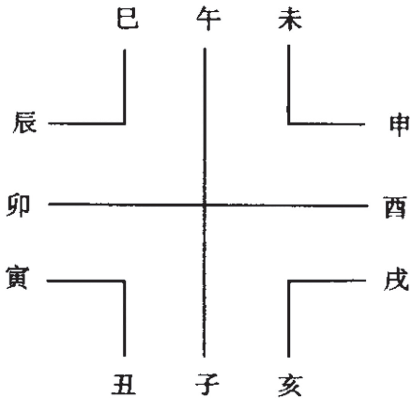
【図四】四仲・四鉤図
