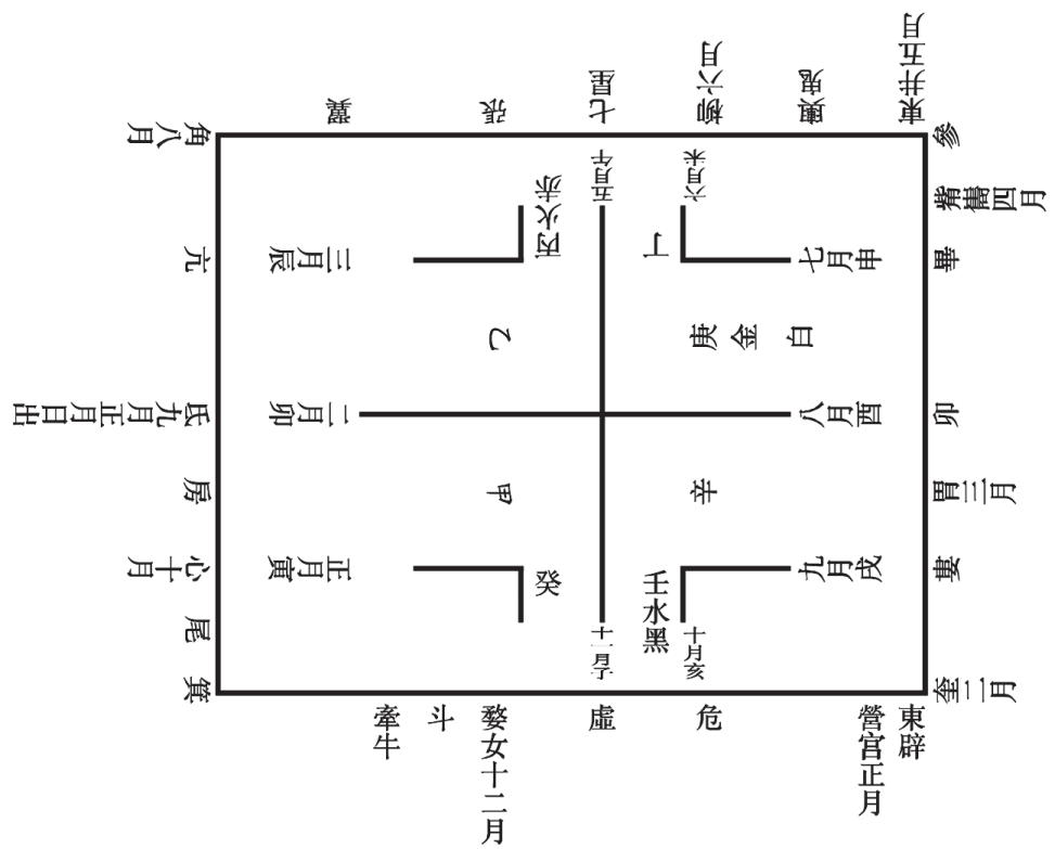
【図六】北大漢簡「日書・式図（甲）」
